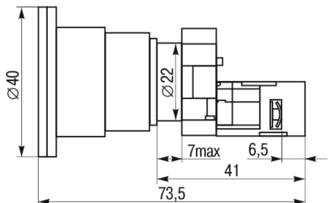
Рисунок 1 (продолжение) - Габаритные и присоединительные размеры кнопок
