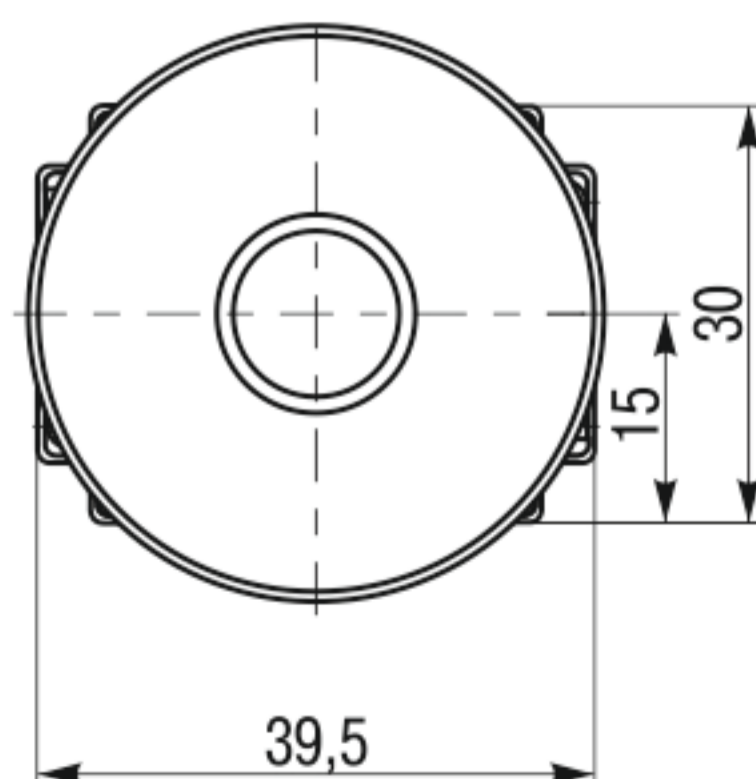
Рисунок 1 (продолжение) - Габаритные и присоединительные размеры кнопок
